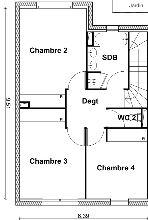
ÉTAGE
