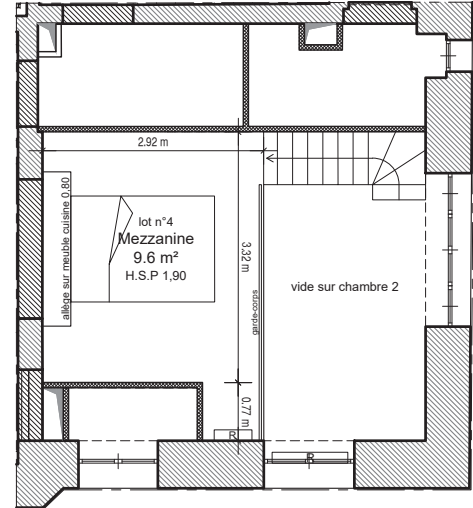
Plan mezzanine chambre 2
