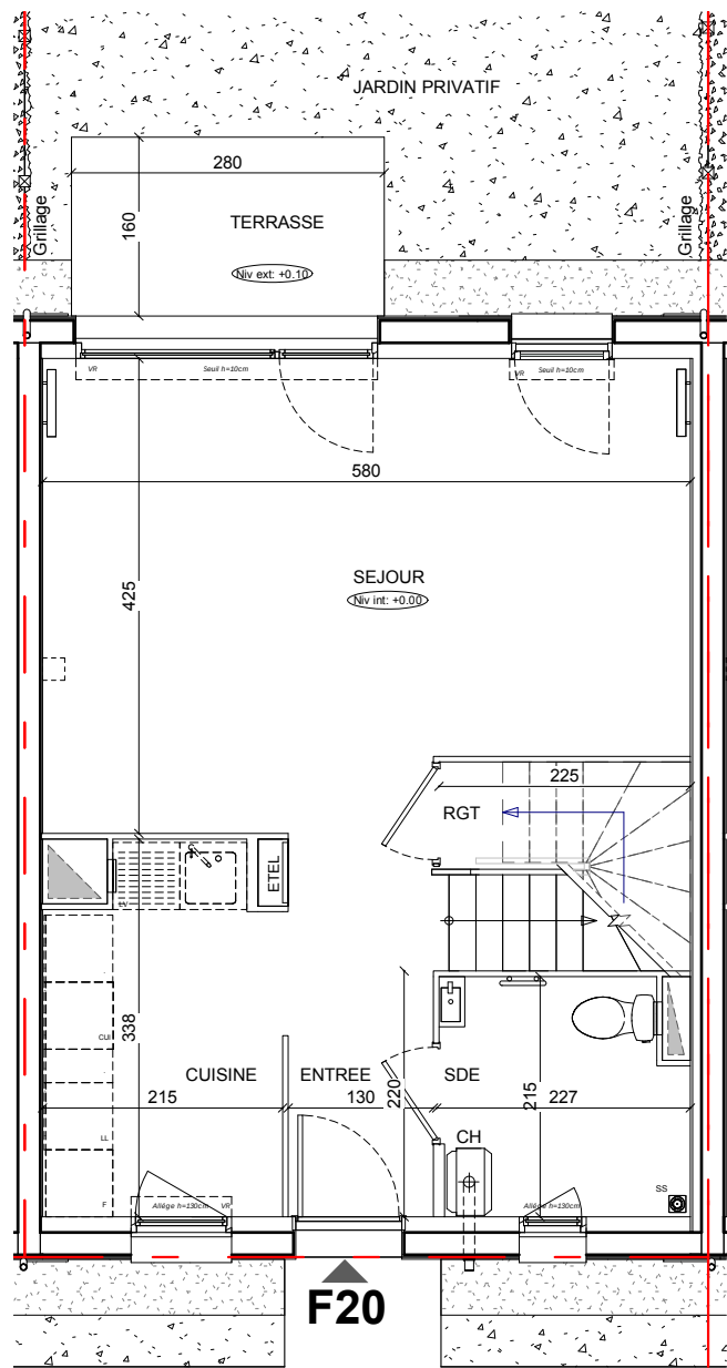
Niveau Bas
