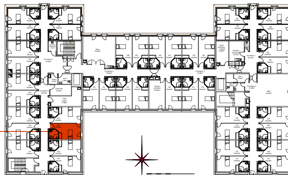
Plan de localisation R+2
