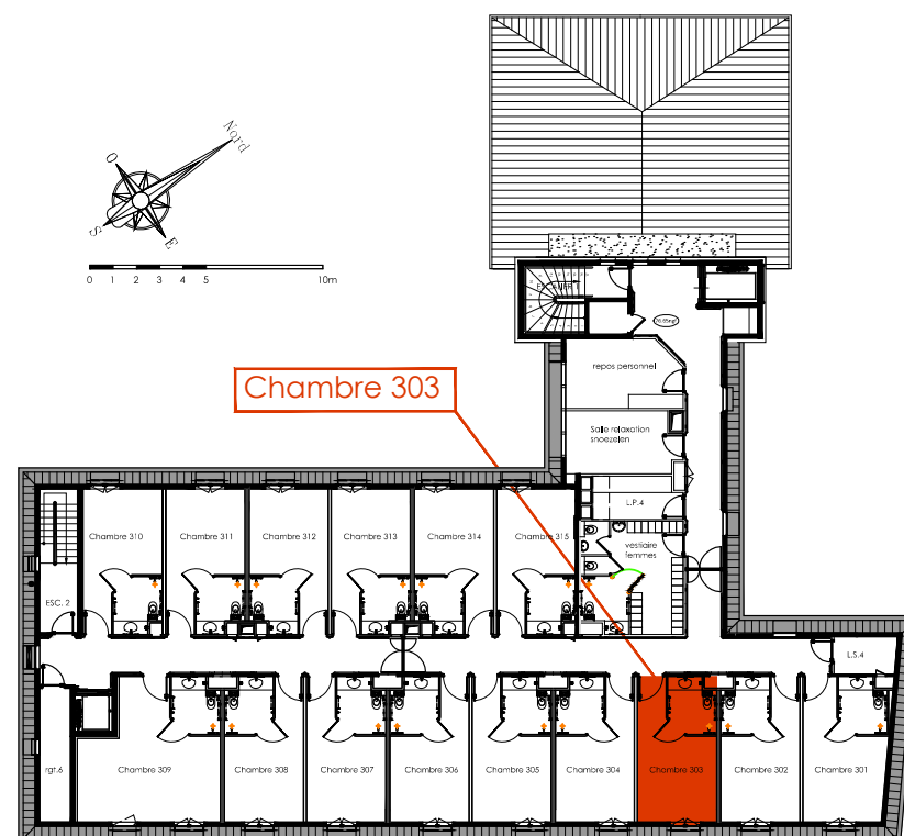
Plan de localisation R+2
