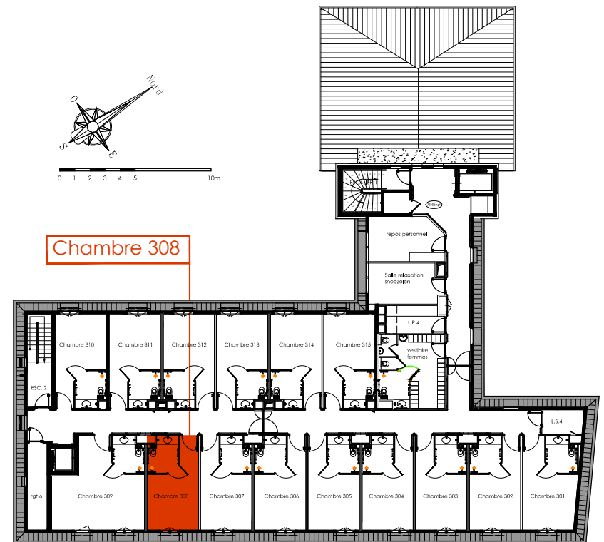
Plan de localisation R+2
